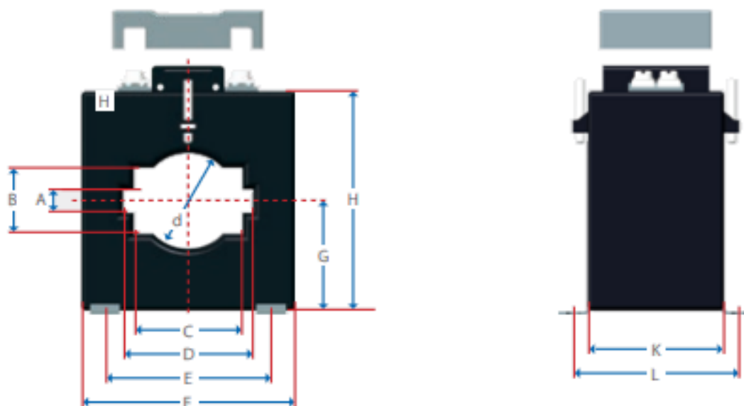
Wymiary [mm]
